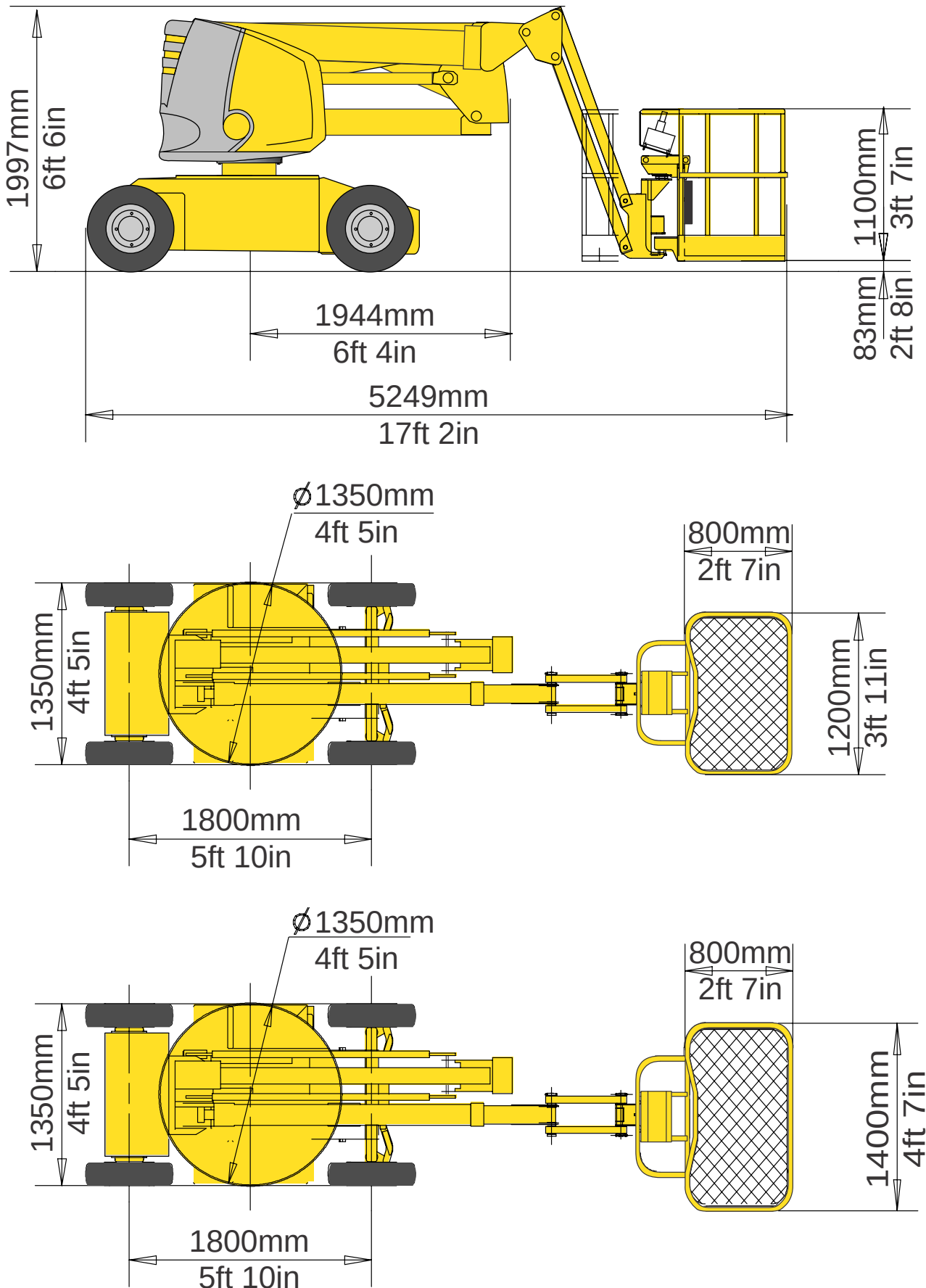
Fig. 4 - Espacio ocupado HA12IP
