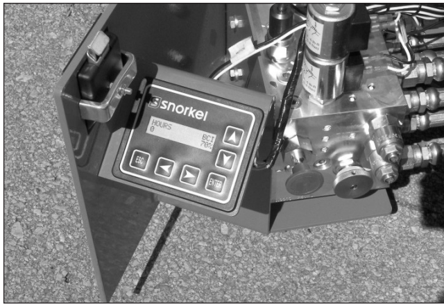
Figura 4 – Pantalla LCD del centro de diagnóstico
