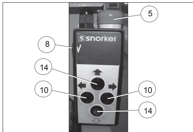
Figura 3: Controles superiores colgantes
